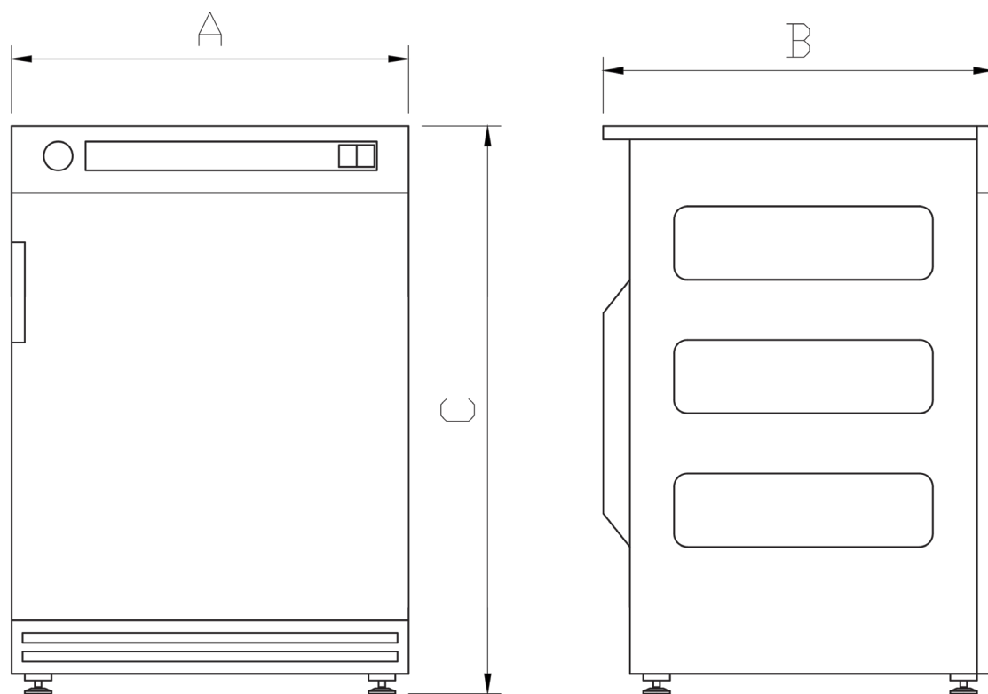
Размеры эскизов
