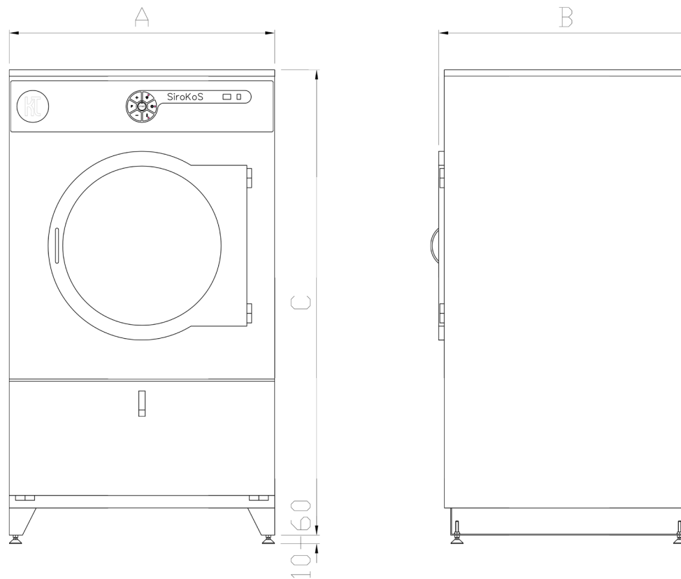
Размеры эскизов
